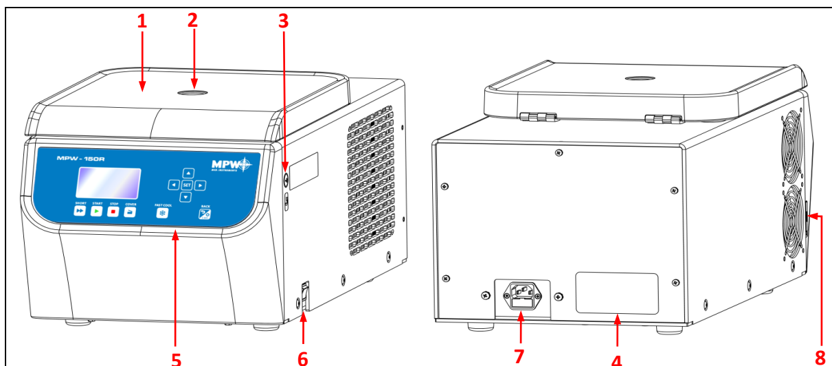
Rys.1. Przód wirówki MPW-150R
