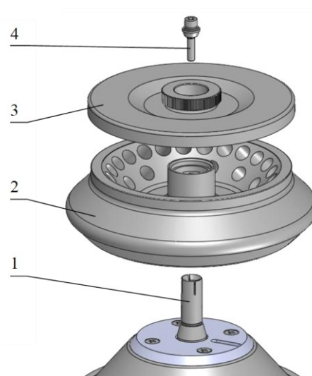
Rys.3. Zespół wirnika kątownego
